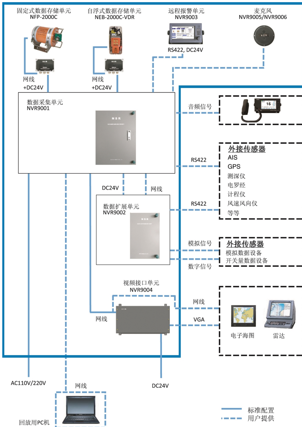
系统框图
