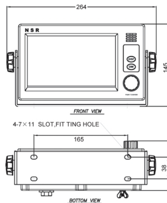
DISPLAY UNIT
